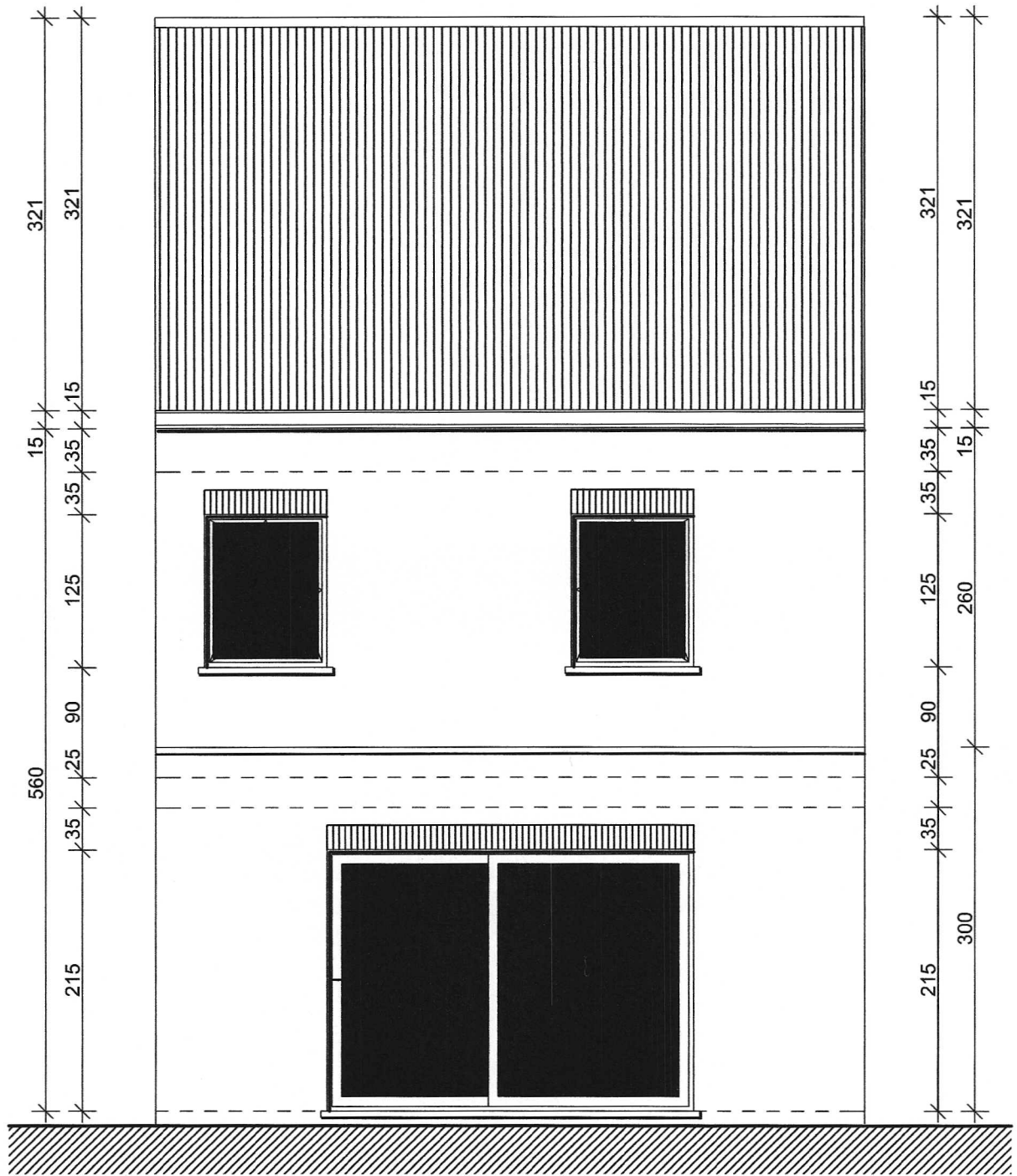
achtergevel
