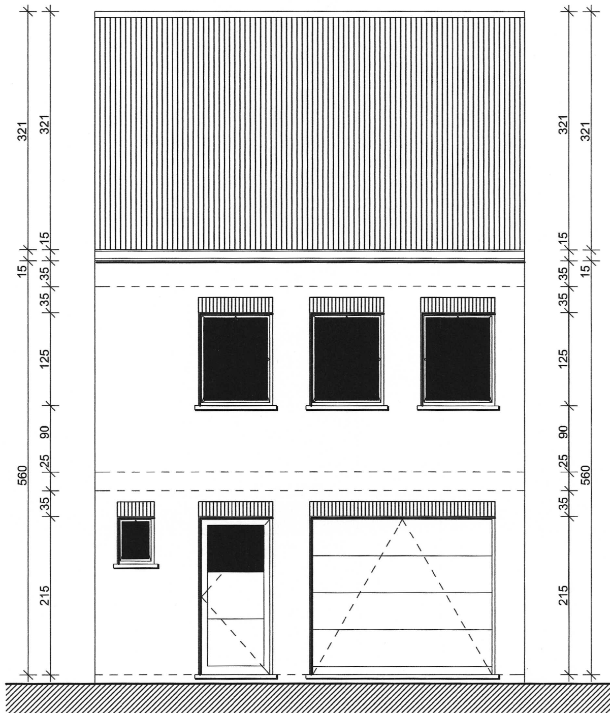
voorgevel
