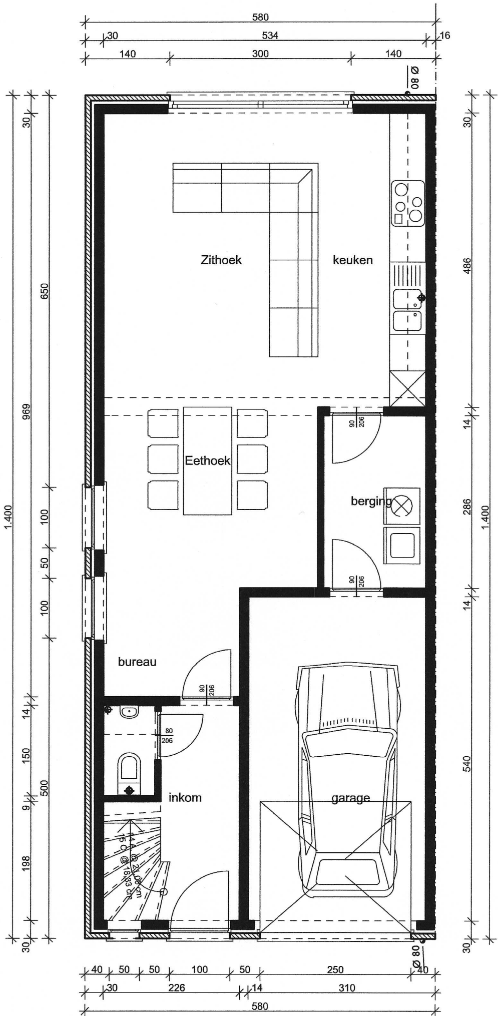
grondplan
